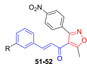
51 , R= -Cl 52 , R= -Br
